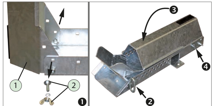
Rabattre la tôle de butée avant vers le bas
