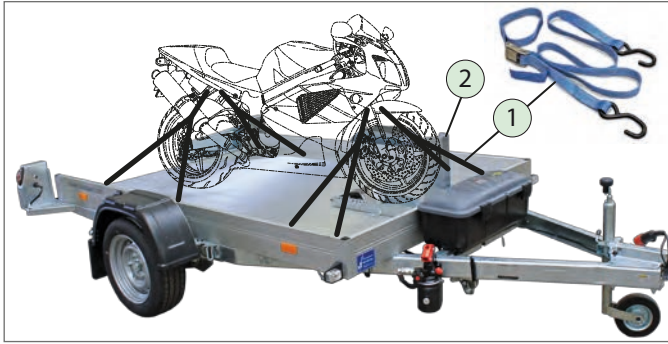
Moto arrimée
