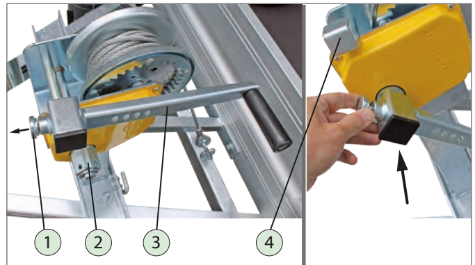
Mise en place de la manivelle
