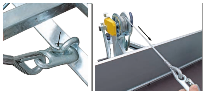
Déroulement du câble
