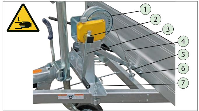
HKT avec treuil à câble
