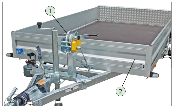
avec treuil à câble & ridelles rehaussées
