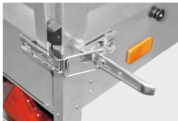
Spansluitingen op de achterklep
