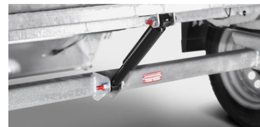
Kantelbare bak (kantelbaar op HA) met schokdemperondersteuning
