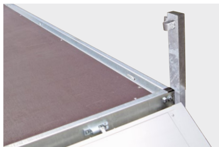
Stanchion pockets en verwijderbare stanchions, beide thermisch verzinkt
