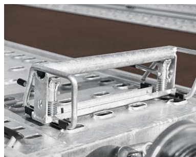
Stabilité particulière grâce aux profilés à double chapeau fixés au pont dans le sens transversal
