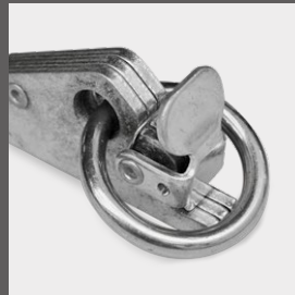
Raccords pour le rail d'arrimage du chargement (4 pièces)
