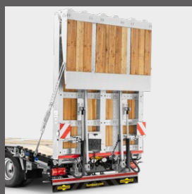
2-delige opritwand over de gehele breedte met houten beplanking houten planken
